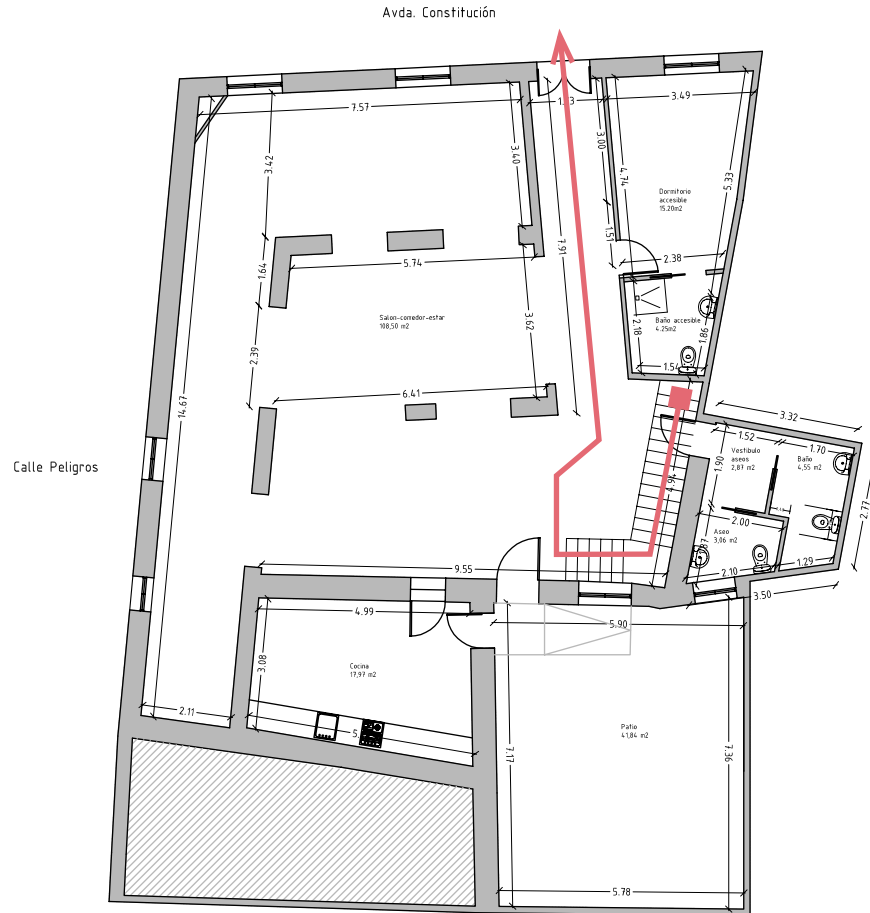
ESTADO REFORMADO PLANTA BAJA
