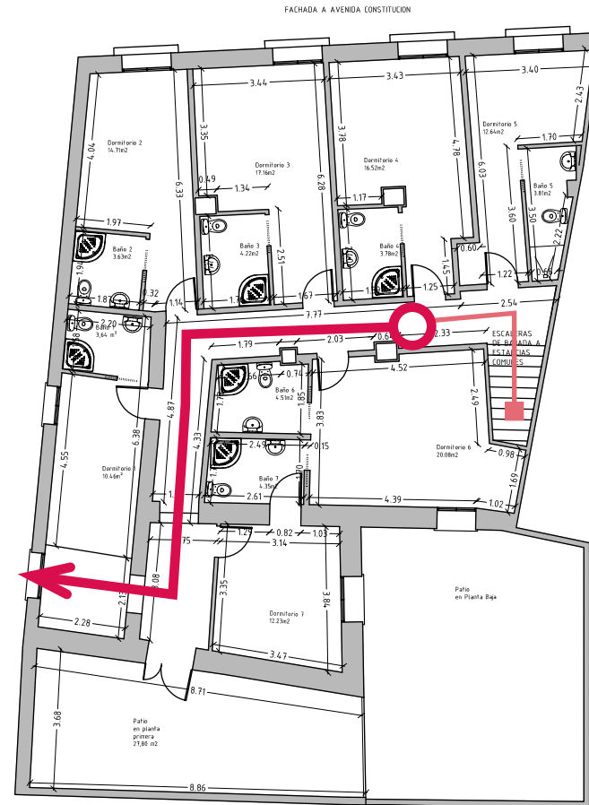
ESTADO REFORMADO PLANTA PRIMERA
